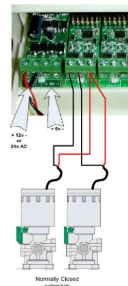
Branchement du Programmeur Filtron
