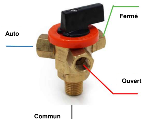
Robinet 3 voies
