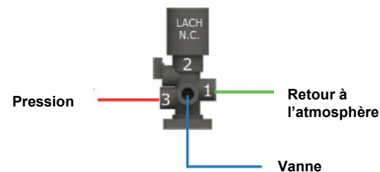
Robinet 3 voies
